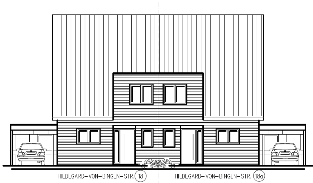
Westansicht
